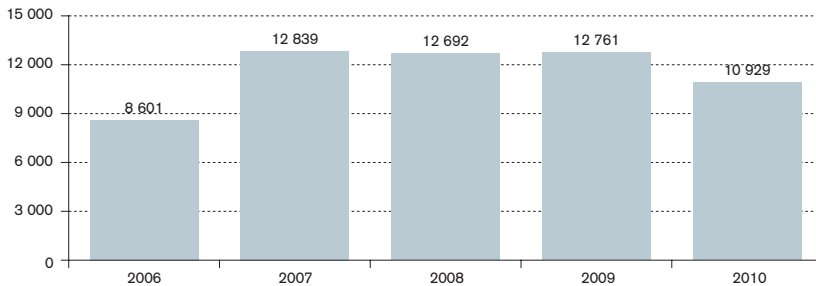
Nombre d'heures de fonctionnement des fours
